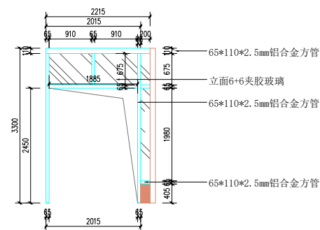
住院部收费大厅斗侧面大样
