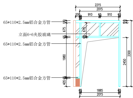
住院部收费大厅斗侧面大样
