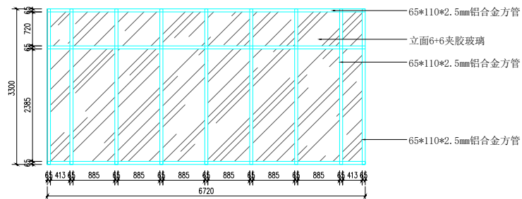
住院部收费大厅斗正立面大样
