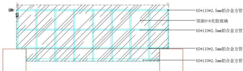
住院部收费大厅斗顶面大样
