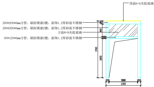
住院部北门斗侧面大样 (外)
