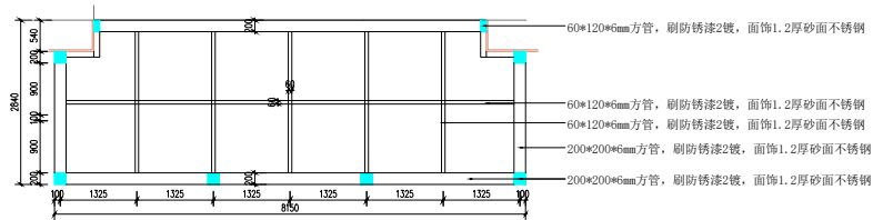
住院部北门斗顶面大样 (外)
