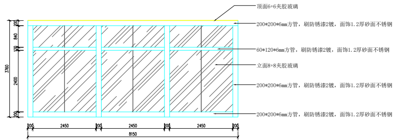
住院部北门斗正立面大样 (外)
